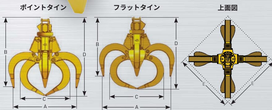
略図の寸法
